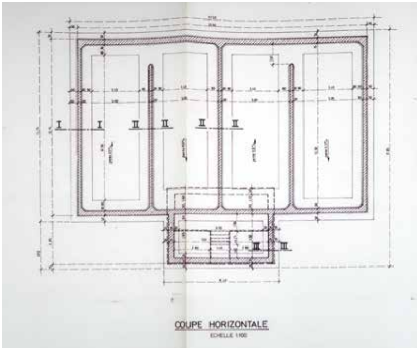
◀ Grundriss des Réservoir Lintgen Ponts et Chaussées, Distribution d'Eau de Lintgen. Construction d'un réservoir d'eau potable de 1 000m 3 avec conduites d'aduction et de refoulement pour la localité de LINTGEN. Coupes horizontales-longitudinales et transversales, [Plan], Gemeinde-archiv Lintgen, Luxemburg, 1974.
