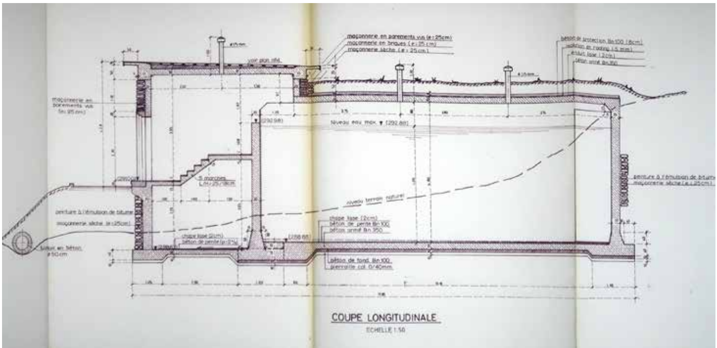
▲ Längsschnitt des Réservoir Lintgen Ponts et Chaussées, Distribution d'Eau de Lintgen. Construction d'un réservoir d'eau potable de 1 000m 3 avec conduites d'aduction et de refoulement pour la localité de LINTGEN. Coupes horizontales-longitudinales et transversales, [Plan], Gemeindearchiv Lintgen, Luxemburg, 1974.
